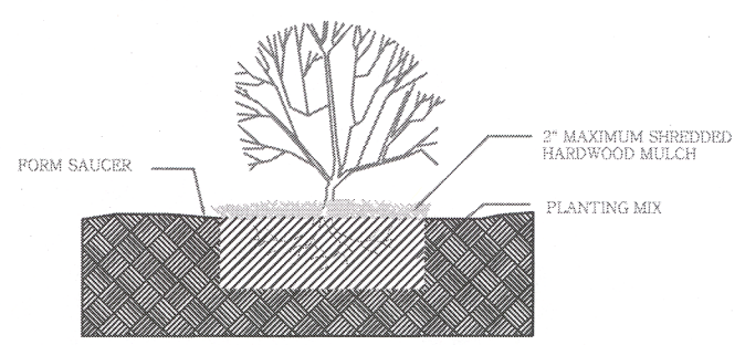
BARE ROOT
